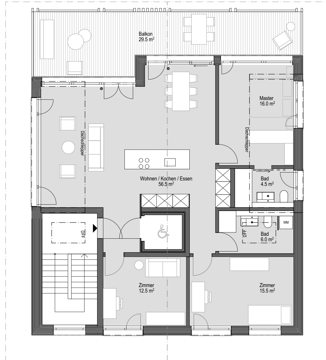
Mst. 1:100
