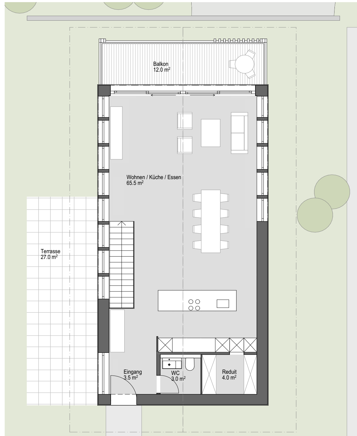
Mst. 1:100
